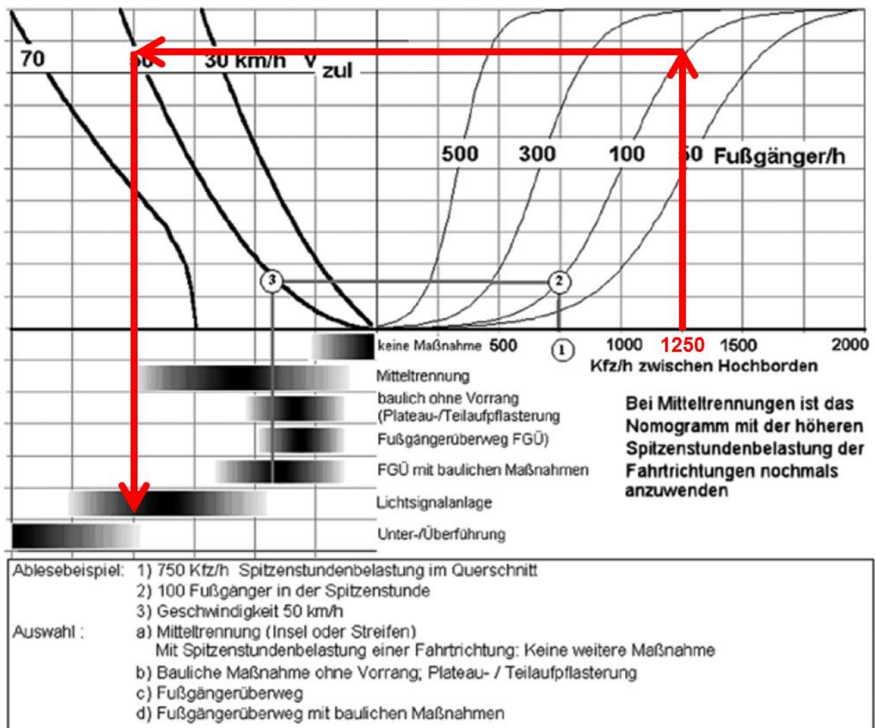
Abbildung 9: Einsatzbereiche von Überquerungsanlagen an zweistreifigen Straßen mit Fahrbahnbreiten unter 8,50 m
